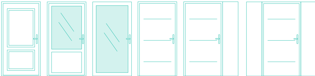
Porte seule 1 vantail
